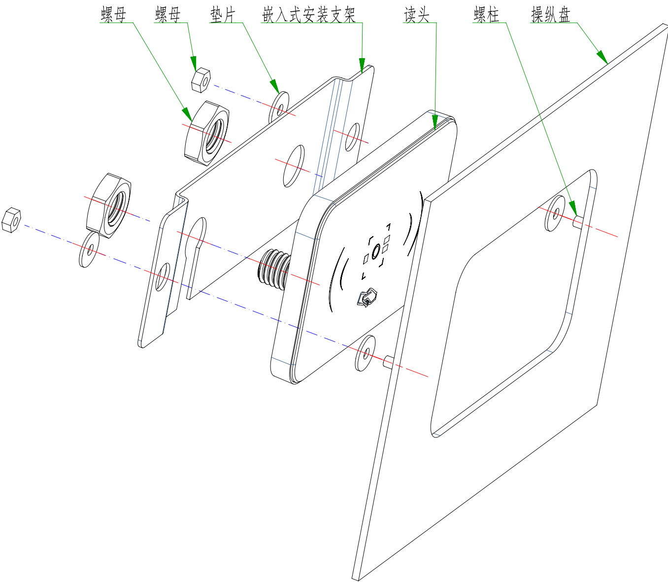
嵌入式安装图解
