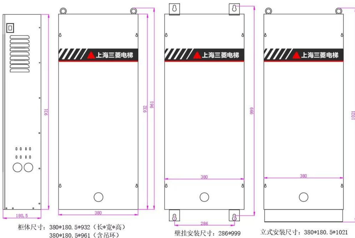
工地安装尺寸图
