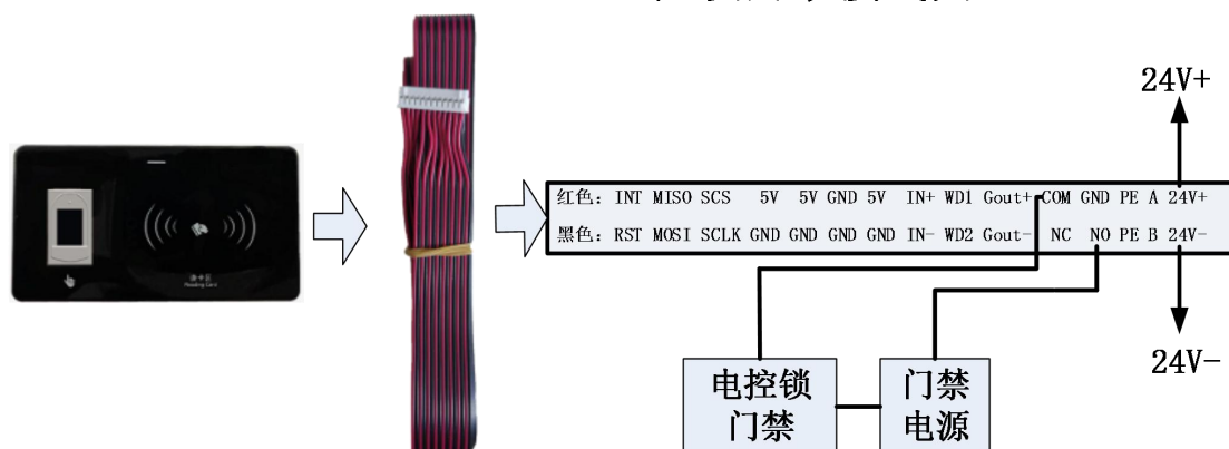
电控锁门禁接线图
