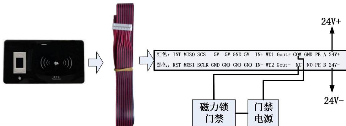
磁力锁门禁接线图
