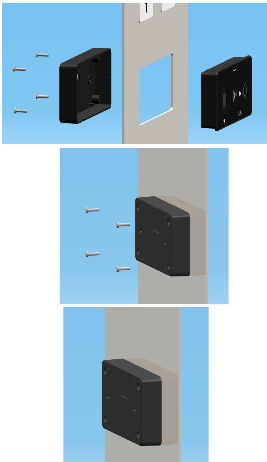
1.3 开孔图
